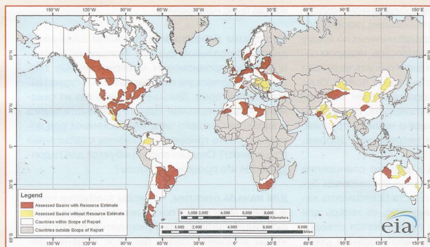
▲ 48 сланцевых бассейнов (выделены коричневым цветом) в 38 странах (выделены белым цветом), включенных в отчет U. S. Energy Information Administration «World Shale Gas Resources: An Initial Assessment of 14 Regions Outside the United States» 2011
